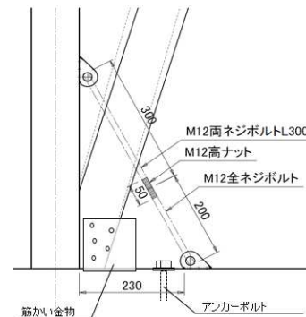
<オリジナル柱頭柱脚金物>
